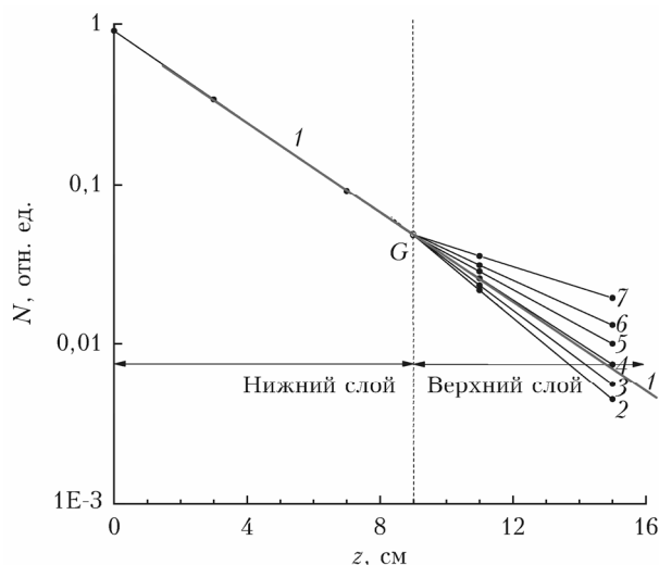
Рис. 1. Нормированные вертикальные распределения концентрации сальтирующих частиц в нижнем (1) и верхнем слое сальтации (2–7) при скоростях ветра в приземном слое атмосферы от 6,0 до 11,0 м/с (G — точка ветвления профилей)
