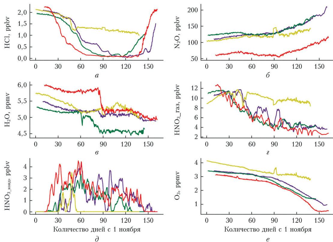
Рис. 2. Вариации отношения смеси HCl ( а ), N 2 O ( б ), H 2 O ( в ), HNO 3_газ ( г ) HNO 3_конд ( д ), O 3 ( е ) в слое 16–25 км, осредненных по ансамблю траекторий: синие кривые — 2010/2011 г., зеленые — 2015/2016 г., желтые — 2018/2019 г., красные — 2019/2020 г.
