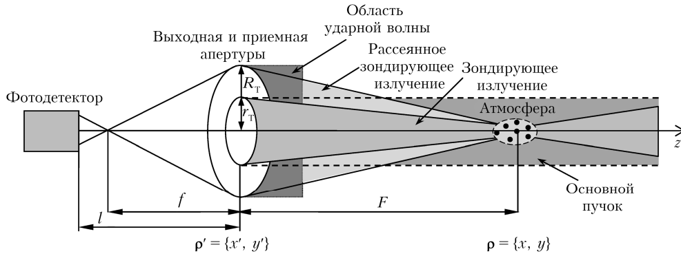
Рис. 1. Упрощенная схема распространения лазерного пучка и приема рассеянного излучения
