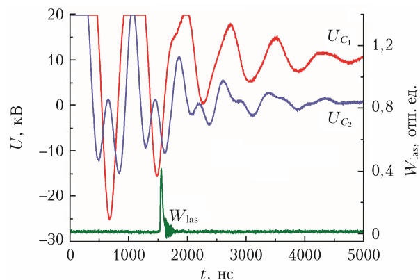
Рис. 2. Осциллограммы импульсов напряжения на емкостях системы накачки C_1 и C_2 и оптического импульса генерации W_{las} пеннинговского индукционного неоновый лазера
