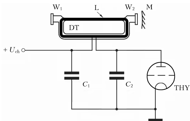
Рис. 1. Электрическая схема системы накачки пеннинговского индукционного неоновый лазера: C_1 = 28,6 нФ; C_2 = 52 нФ; DT — разрядная трубка; L — индуктор-антенна (полужирная линия); ТНУ — тиратрон серии ТПИ1-10к/50; U_{ch} = 27 кВ; W_1 и W_2 — герметизирующие подложки из CaF_2 ; M — зеркало резонатора
