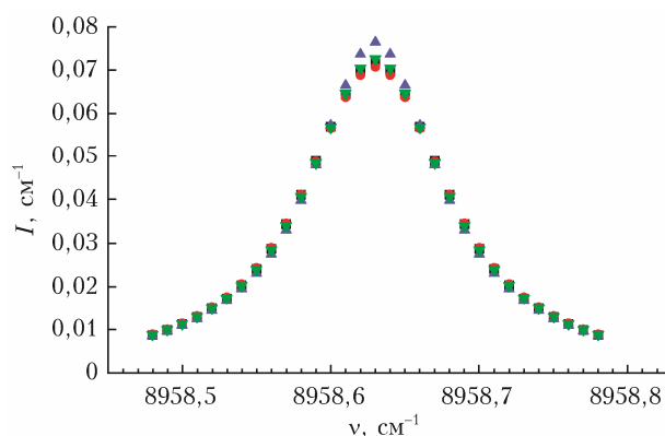
Рис. 1. Контуры линии [9\ 0\ 9] \rightarrow [1\ 0\ 1\ 0] в случае ее уширения Хе: традиционный контур Фойгта, вычисленный с Потенциалами 1 (■) и 2 (●); контур I(\nu) , вычисленный с учетом эффекта ветра по формуле (9) с использованием Потенциалов 1 (▲) и 2 (▼) (см. цв. рис. 1–6 на сайте http://iao.ru/ru/content/vol.37-2024/iss.05 )
