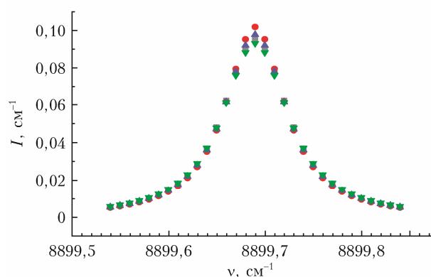
Рис. 2. Контуры линии [4\ 0\ 4] \rightarrow [5\ 0\ 5] в случае ее уширения Аг: традиционный контур Фойгта, вычисленный с Потенциалом 2 (■); контур I(\nu) (9), вычисленный с Потенциалами 1 (●), 2 (▲) и 3 (▼), которые отличаются глубинами потенциальных ям
