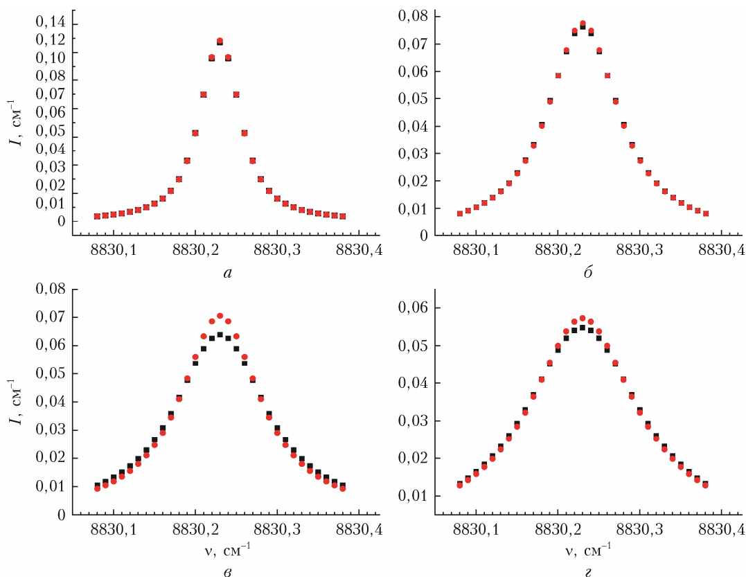
Рис. 3. Контур линии [0\ 0\ 0] \rightarrow [1\ 0\ 1] молекулы \text{H}_2\text{O} полосы \nu_1 + \nu_2 + \nu_3 в случае уширения линии Не (а), Аг (б), Кг (в) и Хе (г), вычисленный с учетом (формула (9)) (●) и без учета эффекта ветра (■)
