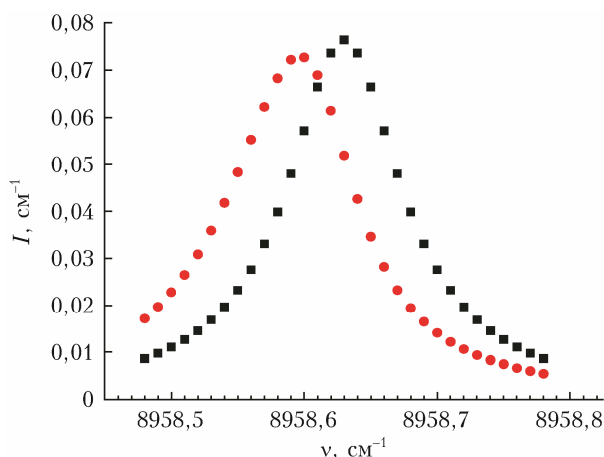
Рис. 6. Контур линии [9\ 0\ 9] \rightarrow [10\ 0\ 10] в случае ее уширения и сдвига Xe, вычисленные без учета (■) и с учетом (●) функции \delta(v_a) из (11)
