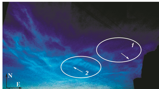
Рис. 3. Атмосферные гравитационные волны в 16:23 UT 25.07.2018 г.: 1 — более длинные, распространяющиеся на северо-восток; 2 — короткие, движущиеся на юго-запад. Эллипсами обозначены группы волн (см. цветной рисунок на сайте http://iao.ru/ru/content/vol.37-2024/iss.05 )
