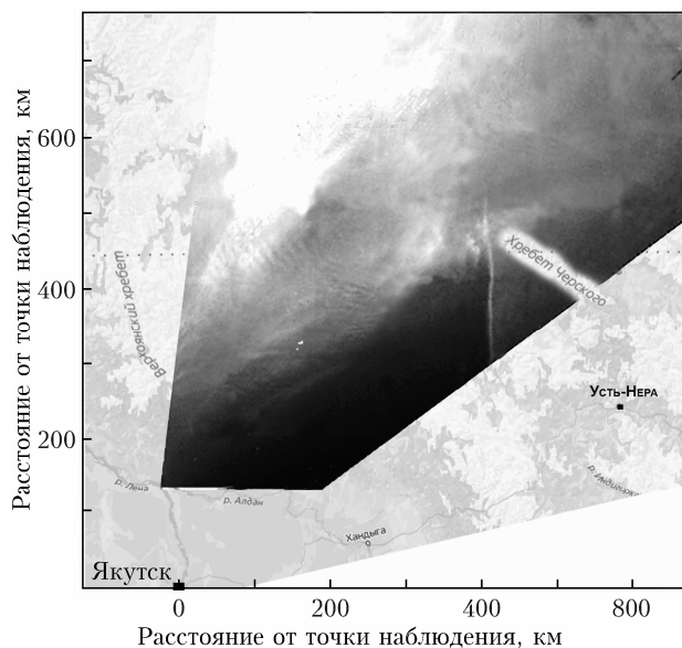
Рис. 2. Проекция рис. 1, a на географическую карту на уровне 79,4 км
