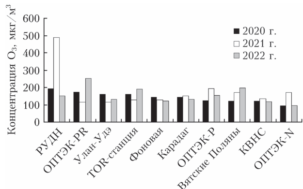
Рис. 5. Годовые максимумы концентрации озона в 2020–2022 гг.
