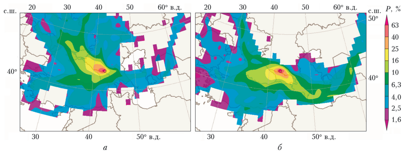
Рис. 7. Вероятность прохождения элементарных воздушных масс, связанных с 10% самых низких (а) и 10% самых высоких (б) аномалий концентрации приземного озона на КВНС в 2022 г., над различными территориями
