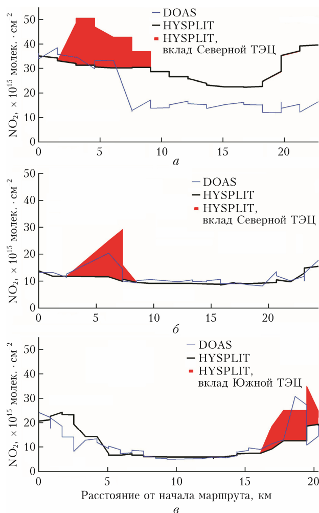
Рис. 4. Содержание \text{NO}_2 на маршрутах 28.03.2016 г. (а), 16.03.2017 г. (б) и 19.04.2023 г. (в) по согласованным по времени данным мобильных измерений (DOAS) и результатам моделирования (HYSPLIT) в точках маршрута с учетом эмиссии ТЭЦ (красная заливка) и без него (черная кривая)
