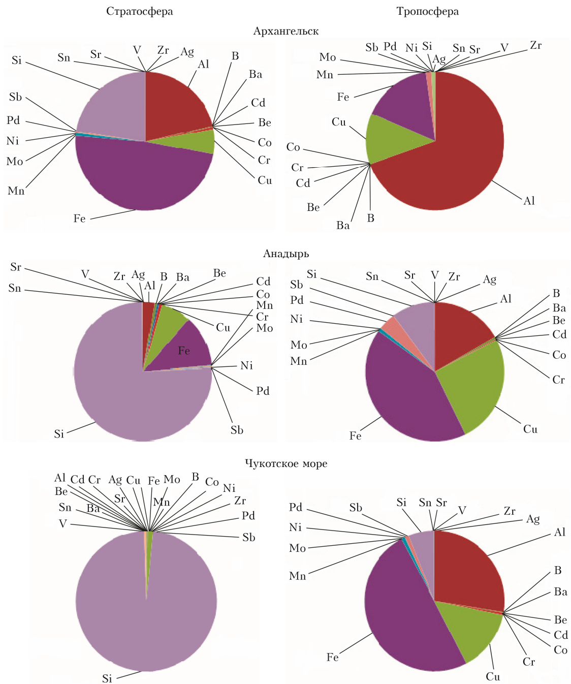
Рис. 5. Элементный состав аэрозоля в стратосфере и тропосфере
