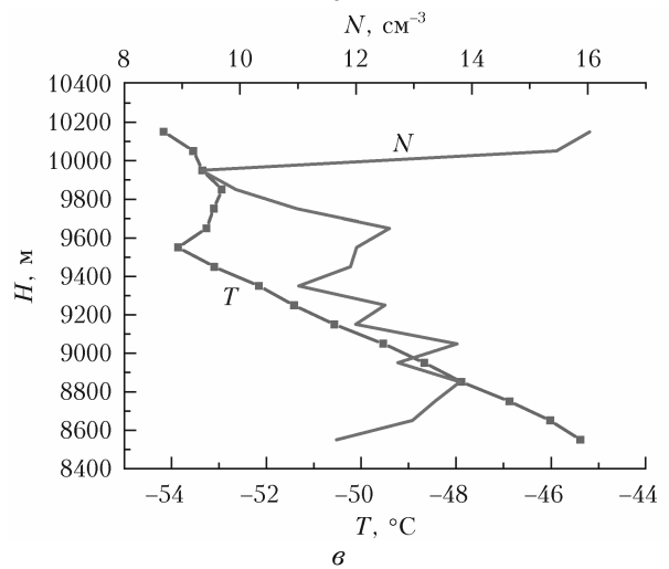
Рис. 3. То же, что на рис. 2, для O 3 (а), NO 2 (б) и счетной концентрации аэрозоля ( d > 0,25 мкм) (в)
