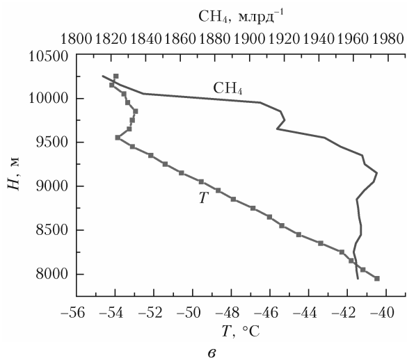
Рис. 2. Вертикальное распределение удельной влажности (а), концентраций CO (б) и CH 4 (в) в слое тропопазузы
