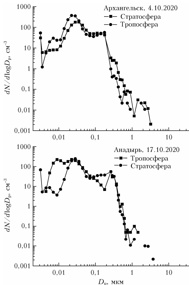
Рис. 7. Распределение частиц аэрозоля по размерам в стратосфере и тропосфере
