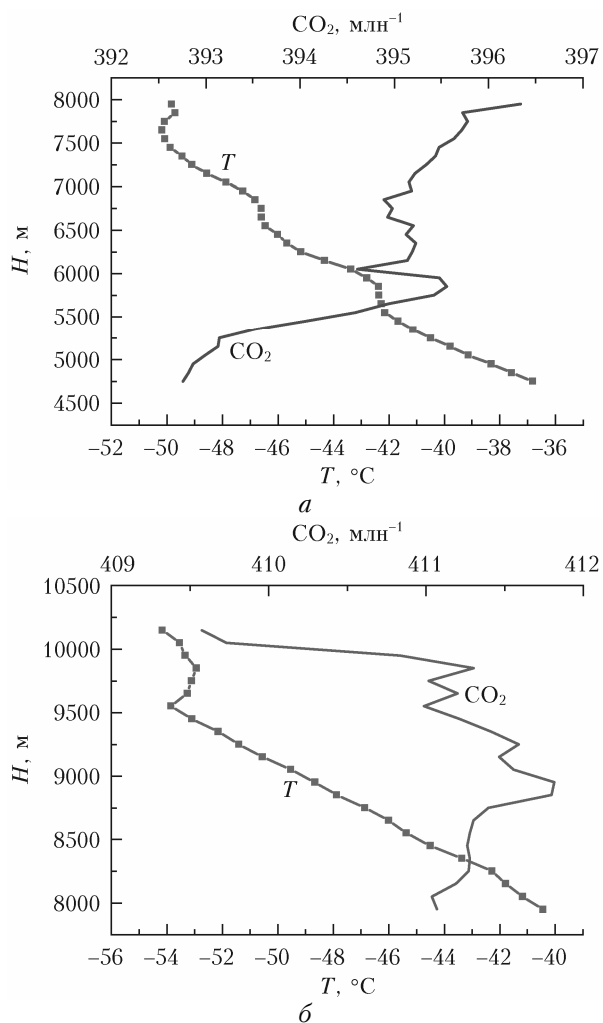
Рис. 4. То же, что на рис. 2, для \text{CO}_2 : a – Карское море, 15.10.2014 г.; б – Архангельск, 4.09.2020
