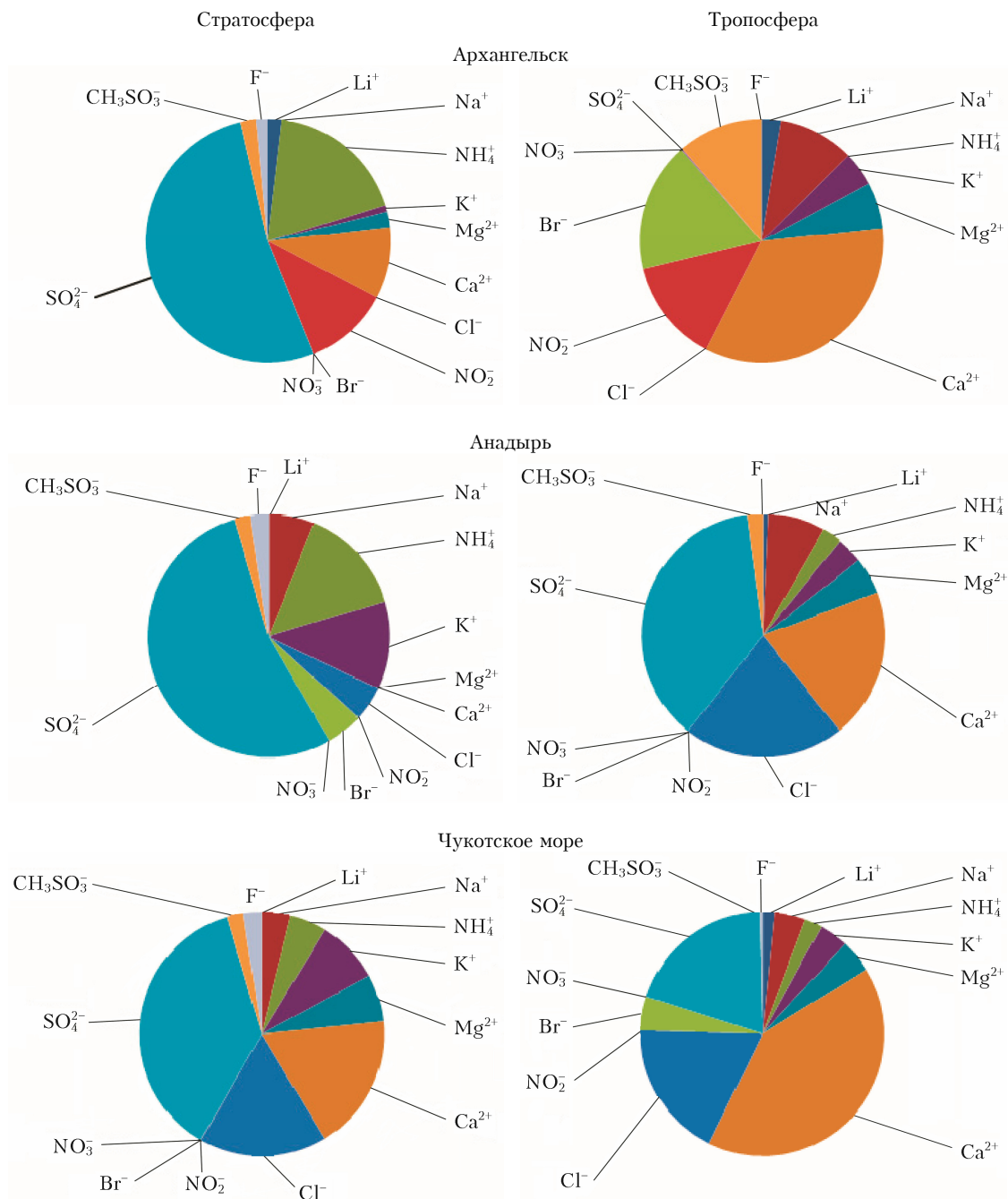
Рис. 6. Ионный состав аэрозоля в стратосфере и тропосфере
