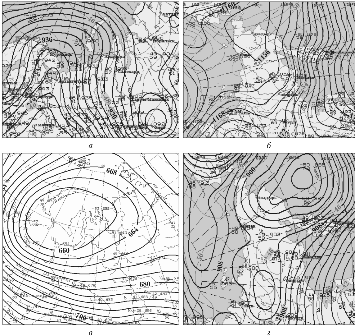
Рис. 1. Карты барической топографии для районов, в которых пересекалась тропопауза (00:00 ВСУ): а – АТ-300, 04.09.2020; б – АТ-200, 17.09.2020; в – АТ-400, 15.10.2014; г – АТ-300, 15.09.2020
