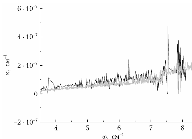
Рис. 3. Континуальное поглощение системы СО: континуальный коэффициент поглощения, извлеченный из эксперимента [13], P_{\text{CO}} = 250 торр (черная кривая); настоящий АТКЛ-расчет с контуром, найденным на основе данных [10–14] (серая кривая). Чистый СО, T = 297 К, P_{\text{CO}} = 250 торр
