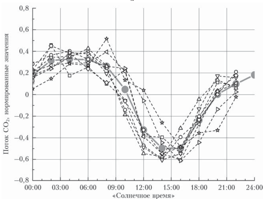
Рис. 4. Нормированный суточный ход парциального давления CO_2 в поверхностной воде (а) и потока CO_2 в системе «вода–атмосфера» (б) в «солнечном времени» для всех месяцев в период открытой воды
