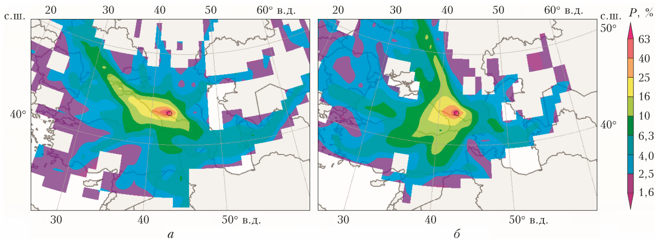
Рис. 4. Вероятность прохождения элементарных воздушных масс, связанных с 10% самых низких (а) и 10% самых высоких (б) аномалий концентрации приземного озона на KBHC в 2023 г., над различными территориями
