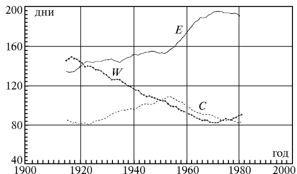
Рис. 3. Сглаженные по 30 годам индексы циркуляции W , E , C . Среднегодовые значения
