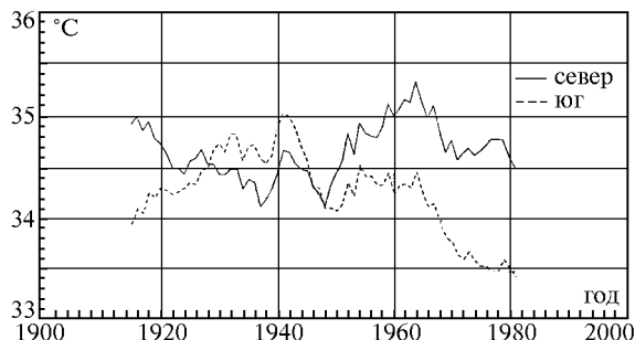
Рис. 4. Сглаженный по 30 годам индекс континентальности
