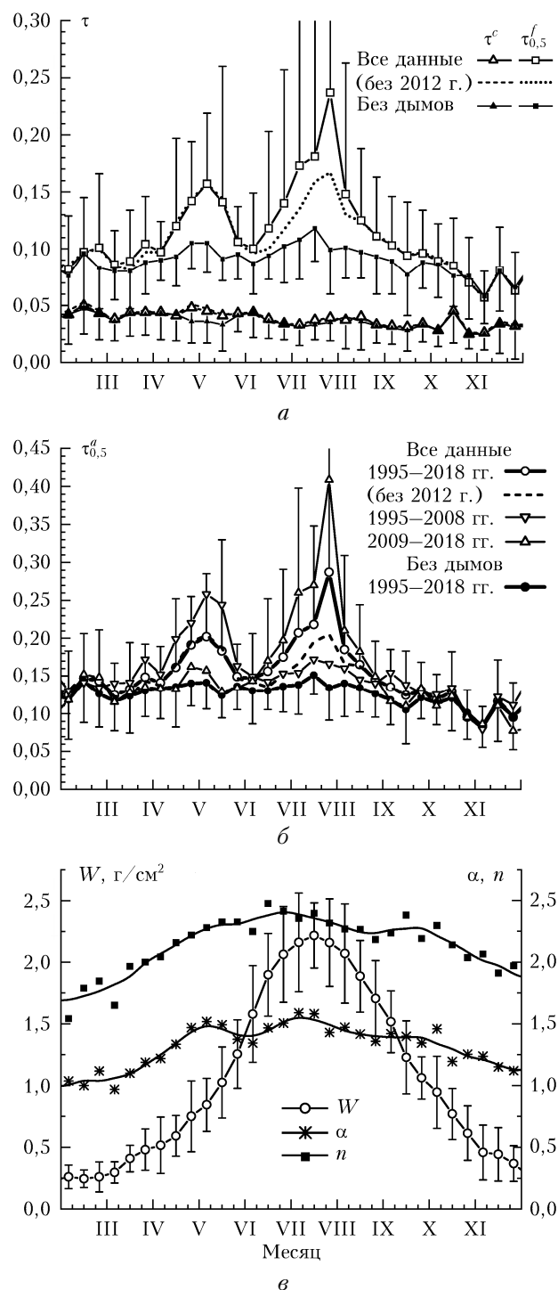
Рис. 2. Годовой ход \tau^c и \tau_{0,5}^f с учетом и без учета дымов (а); \tau_{0,5}^f для разных периодов наблюдений (б); показателей селективности \alpha , n и влагосодержания атмосферы W (в)
