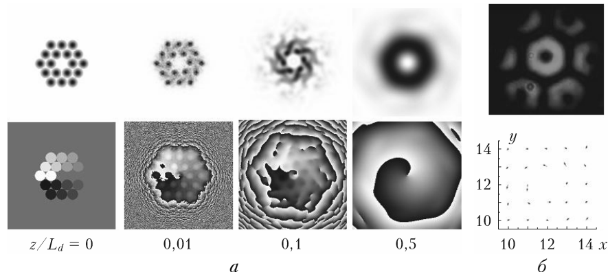
Рис. 3. Результаты: a – численного моделирования; b – лабораторного эксперимента по формированию ОУМ = 1. Верхние рисунки – амплитуда, нижние – фаза излучения (для b – распределение вектора Умова–Пойнтинга)
