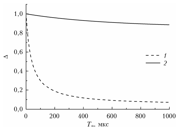
Рис. 3. Доля H_2O в суммарном тепловыделении смеси 1% H_2O и 500 ppm CO_2 в N_2 в зависимости от длительности импульса возбуждающего излучения для двух длин волн, соответствующих линиям генерации CO_2 -лазера 10R(18) (1) и 10R(20) (2)
