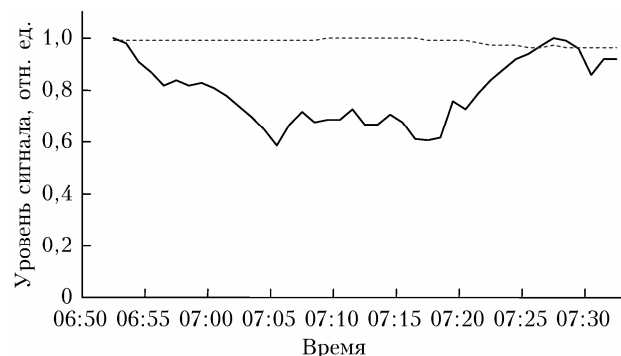
Рис. 3. Изменение уровня сигнала в атмосферном канале при проходе слоя тумана (с МДВ от 0,9 км) на высокогорной трассе 100 м для лазерного излучения на \lambda = 1,55 мкм (сплошная кривая) и миллиметрового излучения на \lambda = 4 мм (штриховая кривая)
